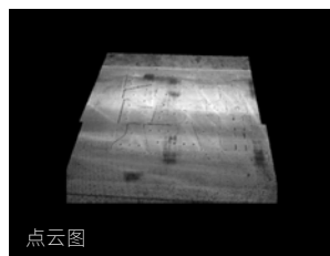
缝隙较小、规格多样的切割钢板
