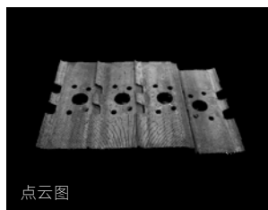
履带板
